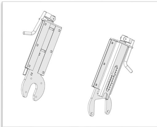
Wellenführung Lagerseitig
