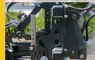
Attelage aux grues agricoles avec compensation de niveau et béquille de support.
