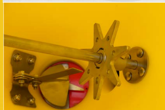
L'agitateur-batteur développé par ADLER évite que le produit d'épandage ne forme des ponts.
